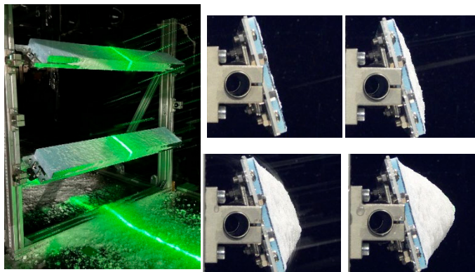
模擬板への着雪実験(左)と時々刻々の着雪形状の変化(右)
