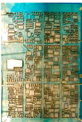
建物の影響を考慮した都市氾濫現象の実験（左）及び松江市を対象とした浸水深のシミュレーション結果（上）
