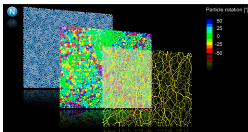
図-2 粒状体のミクロ-マクロ挙動のシミュレーション
