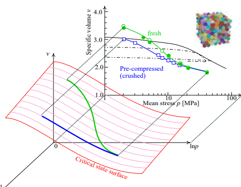
図-1 粒度特性の刻々の変化を巧みに記述した3次元の限界状態面
