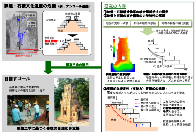
アンコール遺跡 (カンボジア) を対象とした安定性評価手法の開発とその応用
