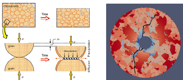
THMCの概念と水圧破碎による解析例
