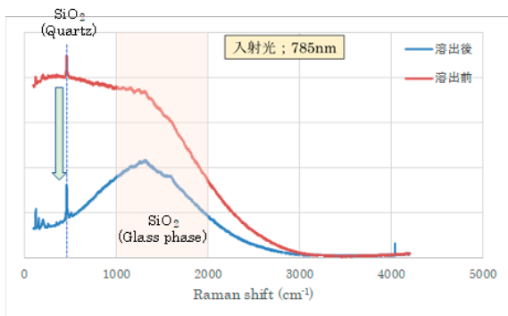
図-1 溶出に伴う骨材のラマンスペクトルの変化
