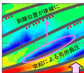
スパイラル状突起間の圧力分布
