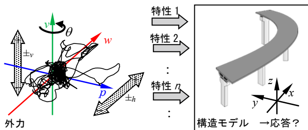
時空間的な方向特性変動に対する応答変動の評価
