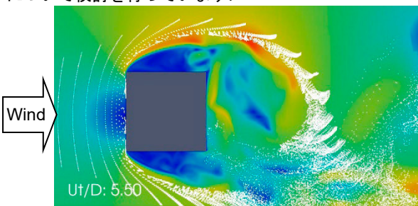
矩形断面周りの粒子飛散解析 (カラーは風速絶対値)
