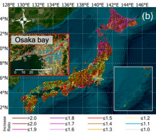
100年に1回の洪水の将来変化
