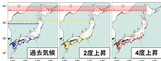
気候モデルシミュレーションによる梅雨豪雨の発生場所
