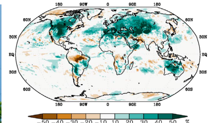
夏季降水量に対する農地灌漑の影響。
