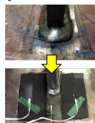
接着補修後の残存疲労寿命評価
