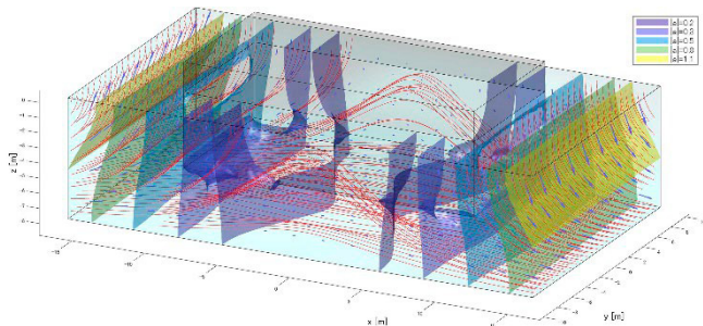
浮体式免震システムの特性評価
