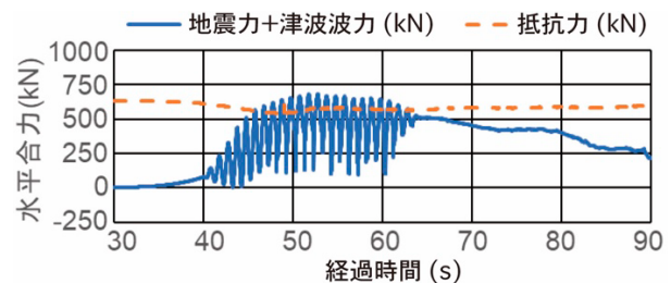
防波堤に作用する水平方向合力の時刻歴
