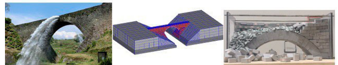
図3 石造アーチ橋と数値解析モデル、振動台実験結果の一例
