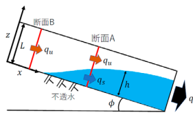
斜面の水の流れのモデル化
