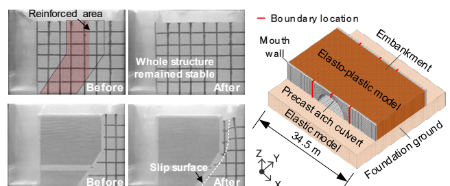
補強領域に着目した遠心実験
