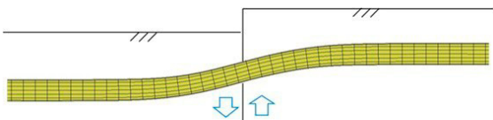
図1 断層を跨ぐ埋設管の数値解析
