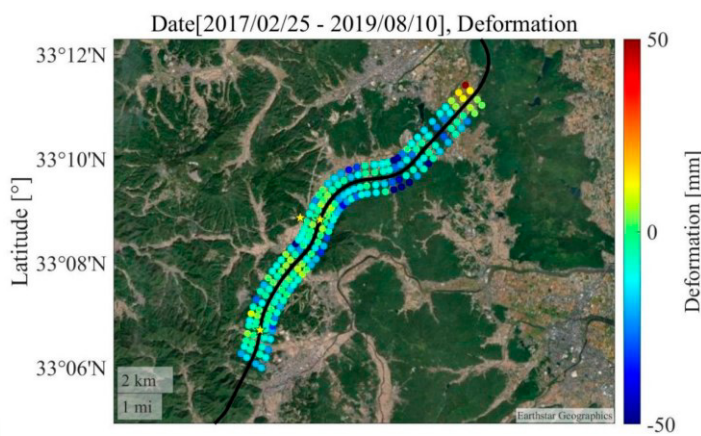
衛星 SAR 画像解析による高速道路周辺の鉛直変動量の分布図。2019 年 8 月 28 日に高速道路周辺で土砂災害が発生し、高速道路路面も変状が発生しました。解析結果の青色で示される箇所はより沈下量大きいことを示しています。
