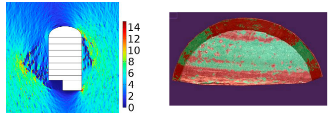
損傷理論を用いた地下空洞掘削解析
