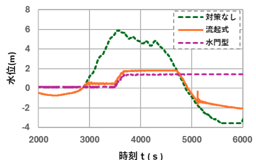
流起式可動防波堤の津波低減効果
