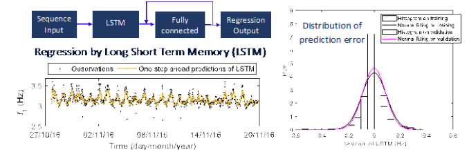
図4. 深層学習による季節変動の予測と予測誤差分布
