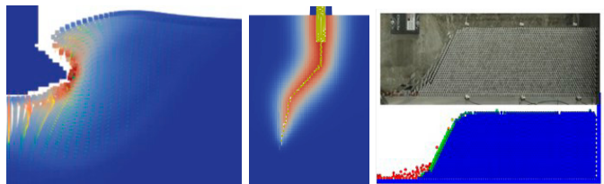
スパッドカン貫入 (MPM), 透水岩盤の水圧破碎 (PD), 岩盤斜面模型の振動解析 (DDA)
