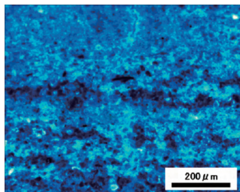
図3 シェールガス・オイルの貯留岩として注目されているシェール(頁岩) 中の間隙構造の評価 (白色部が可視化された微小な間隙)
