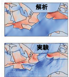
引張変形時の結晶粒内ひずみ分布の予測
