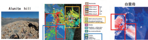
ハイパースペクトル衛星データ (HISUI) を用いたアメリカCuprite地区の鉱物分布推定結果 現地Alunite hillの様子と空機搭載型センサおよび現地測定で確認されている詳細鉱物分布図 (左)、 HISUI画像を用いた端成分抽出による白雲母 (muscovite) の分布推定結果 (右)
