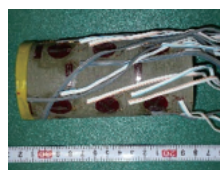
図2 応力計測に用いた岩石コア試料
