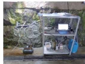
図3 原位置透水試験装置
