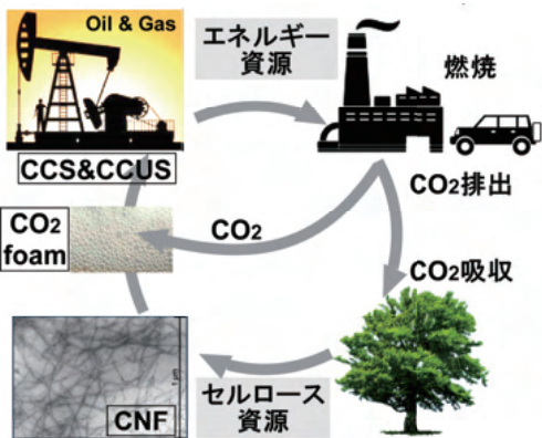
CNF含有フォームによる石油天然ガス開発のカーボンニュートラル化
