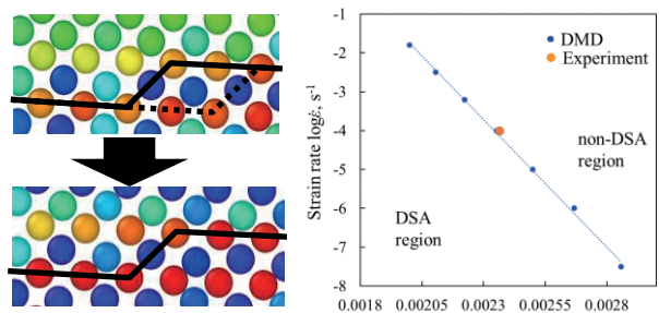
双晶変形に伴う溶質濃度の変化 ひずみ時効の予測
