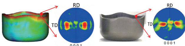
カップ成形性の予測(左:解析, 右:実験)
