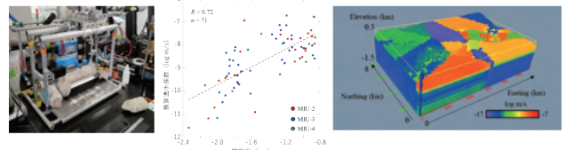
プローブ型パーミアメーター (左) による浸透率測定結果から求めたボーリングコアサンプルの透水系 数と間隙率の比較 (中央) および得られた関係式に基づいて推定された広域地下水構造モデル (右)
