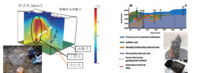
カルデラ構造内部を対象とした熱水流動シミュレーション結果とインドネシア地熱地域でのサンプリング作業の様子 海底熱水鉱床周辺を対象とした変質鉱物分布モデルに基づく熱流体流動パ スの推定結果と海底熱水鉱床のサンプル
