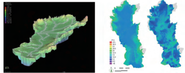
京都盆地の水理地質モデルの鳥瞰図 (左) と土地利用を考慮しない場合の地下温度分布 (中央) 土地利用を考慮した場合の地下温度分布 (右)
