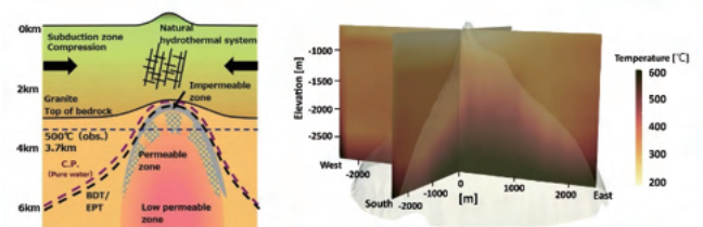
図4 深部地熱システムの概念図(左)、葛根田地熱地域で推定された温度分布(右)
