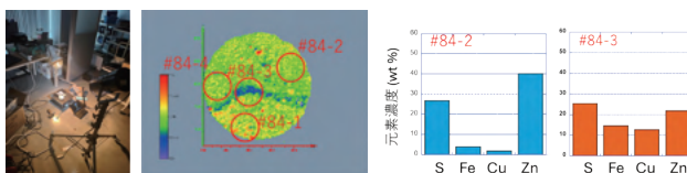
マルチスペクトルカメラによるボーリングコアサンプル断面の撮影とバンド比指数分布 (左・中央) XRFによる元素濃度分析結果 (右) との比較から、Fe, Cu, Znの含有量に対応していることがわかる
